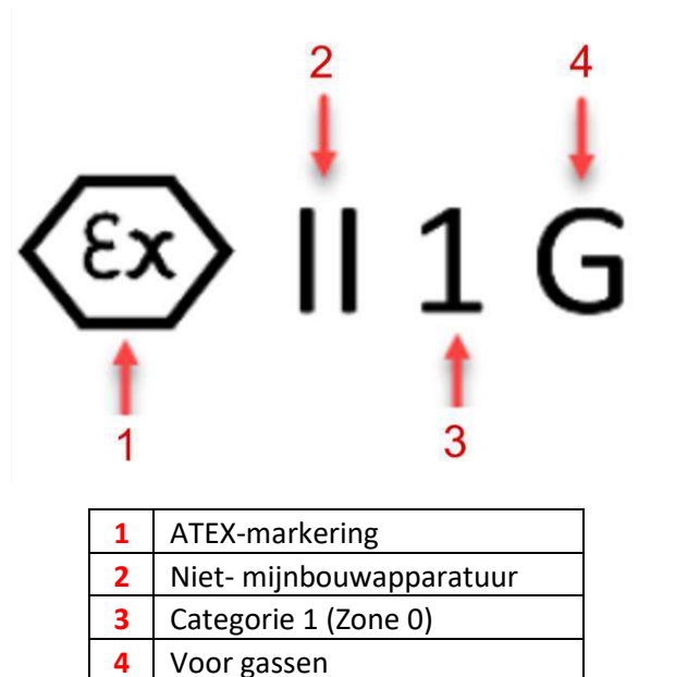
Figuur 2: Beschrijving IECEx explosieclassificatie
