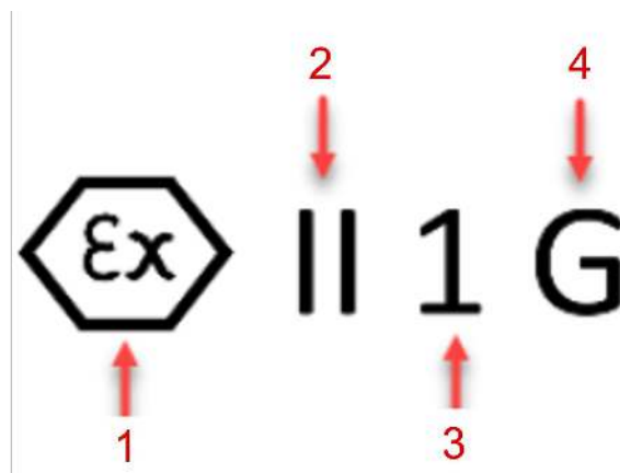
Obrázek 2: Popis klasifikace výbušnosti IECEx
