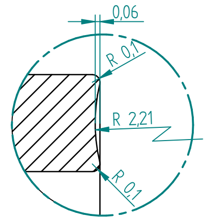
EINZELHEIT B 20:1
